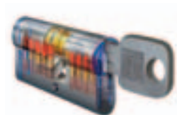
Cylindre Européen à piston
